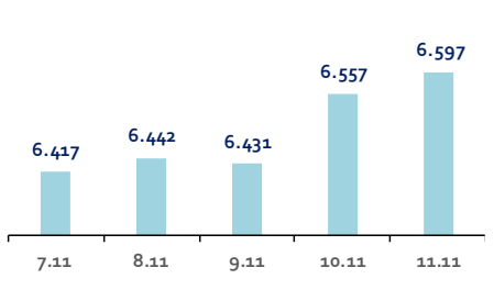
Fransa-CAC40
