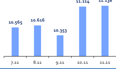
ABD-NASDAQ
