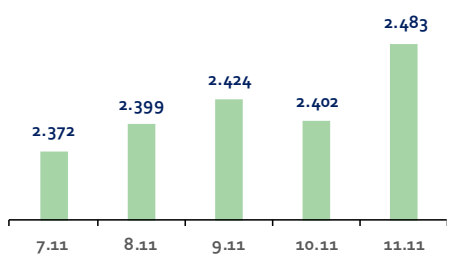
G. Kore-KOSPI
