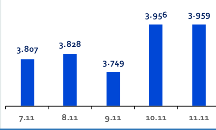
ABD-S&P500
