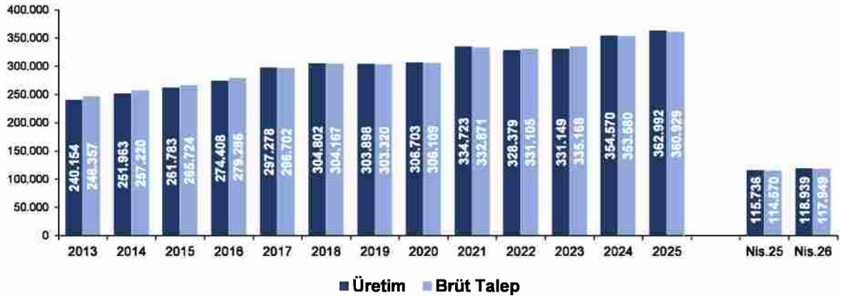
Türkiye Brüt Elektrik Enerjisi Üretimi ve Brüt Talep Gelişimi (GWh)
